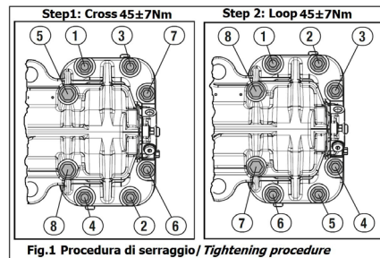
Fig.1 Procedura di serraggio/ Tightening procedure
