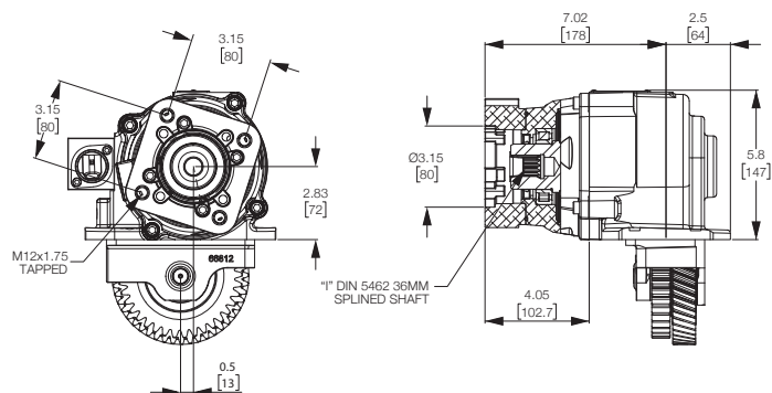
II OUTPUT — DIN 5462
